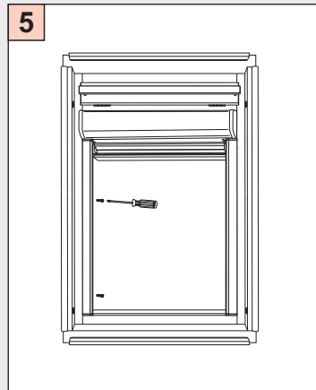
Führungsschienen montage
