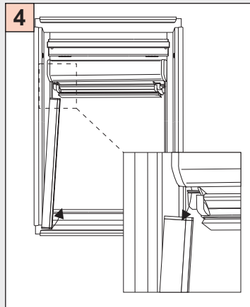
Positionierung der Führungsschienen
