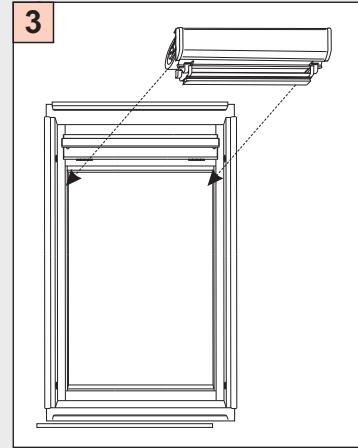
Kassettenmontage
